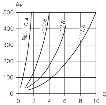
Q 유량 (lpm); Δp 유동 저항 (bar)
