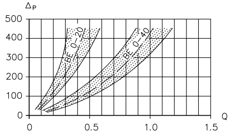
Q 유량 (lpm); Δp 유동 저항 (bar)
