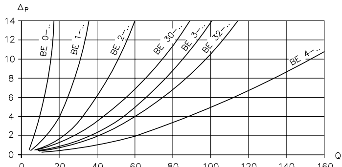
Q 유량 (lpm); Δp 유동 저항 (bar)
