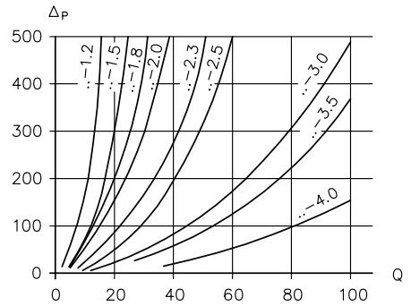
Q 유량 (lpm); Δp 유동 저항 (bar)
