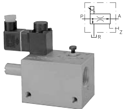
带先导式测流孔的结构形式 如：型号SEHF 3 - 4/70 F - G24
