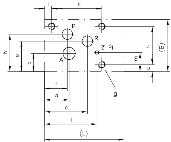
SE 3-3/..和SE 3-4/...型 三通调速阀的板接尺寸
