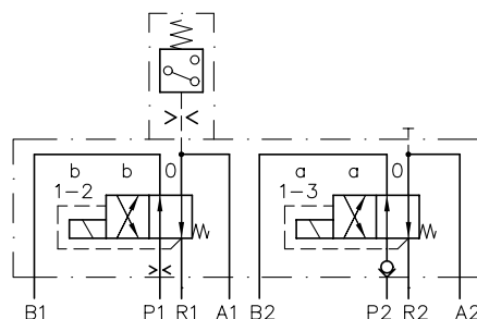
Modelo VZP1W 4 B0,8 WX 2 - WG 110
