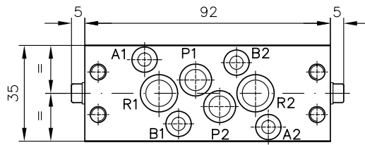
Modelo VZP1 W.. W.-.. 2 válvulas de corredera de 4/2 vías
