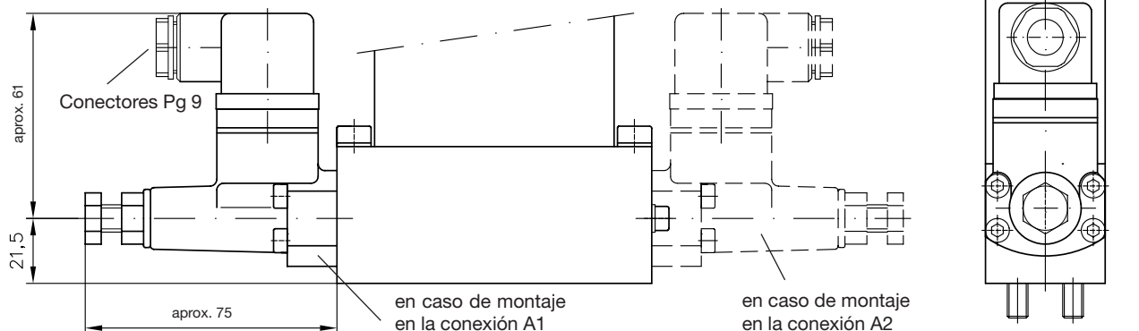
Versión con presostato (datos no especificados, véase catálogo D 5440)
