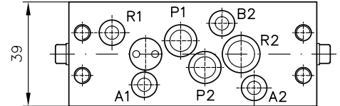
Modelo VZP1 H.. W.-.. ect. Combinación de electroválvula de asiento de 3/2 vías y válvula de corredera de 4/2 vías ¡Las medidas no especificadas corresponden a las medidas indicadas al lado!
