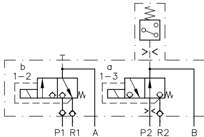
Modelo VZP1H 3 B0,8 F 2 - G 24
