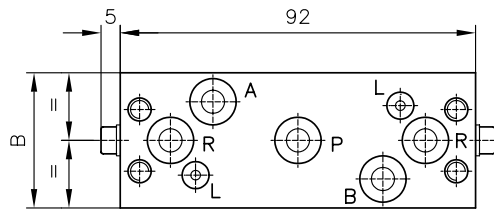
Modelo VZP1 E, G, D y O
