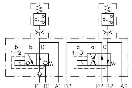
Modelo VZP1R 4 W 4 - G 12
