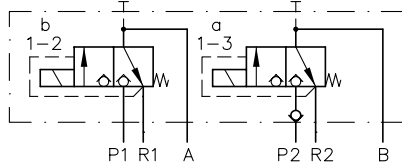
Modelo VZP1N1 2 M1 4 B1,2 - WG 230
