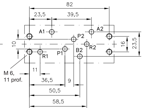
para modelo VZP 1 H.. W.-..
